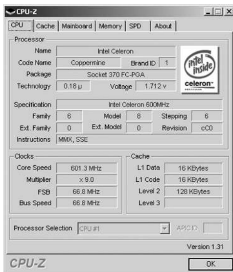
Рис. 8.12. Показания утилиты CPU-Z до разгона процессора Celeron 600 МГц
