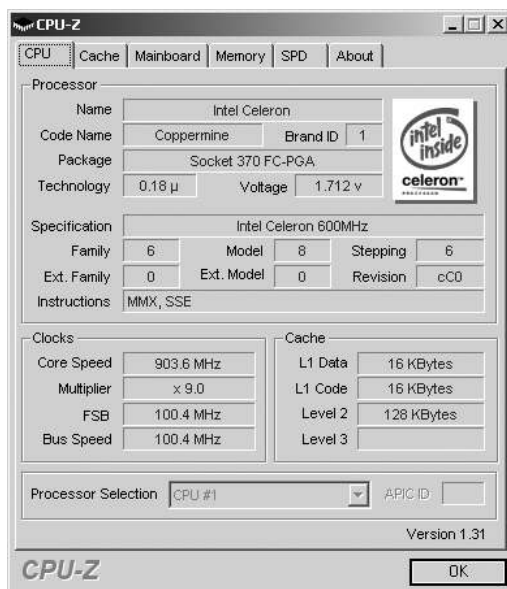
Рис. 8.13. Показания утилиты CPU-Z после разгона процессора Celeron 600 МГц до 900 МГц
