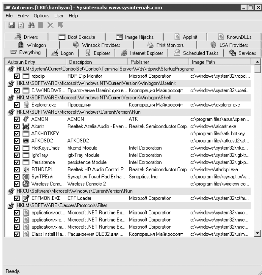
Рис. 9.7. Утилита Autoruns
