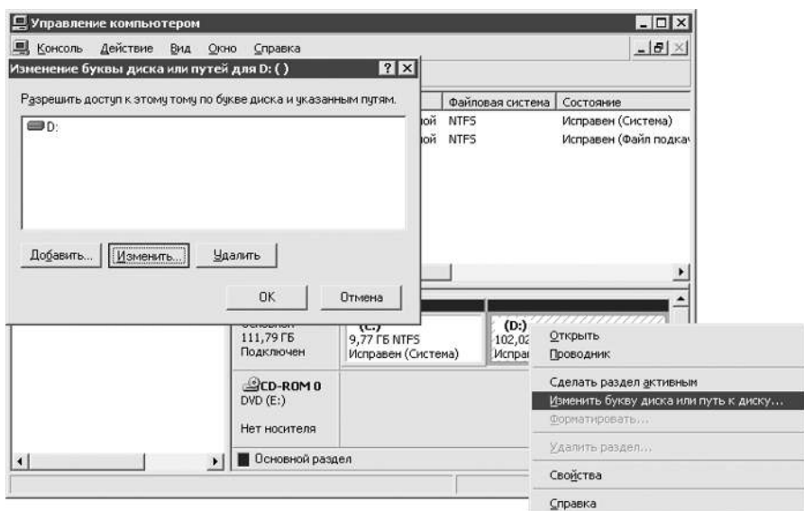
Рис. 9.20. Управление дисками
