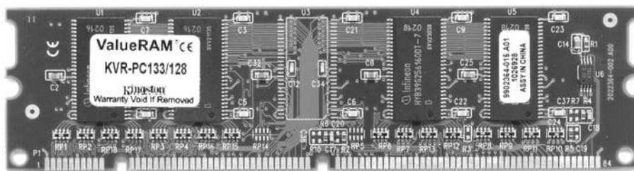
Рис. 2.5. Модуль оперативной памяти
